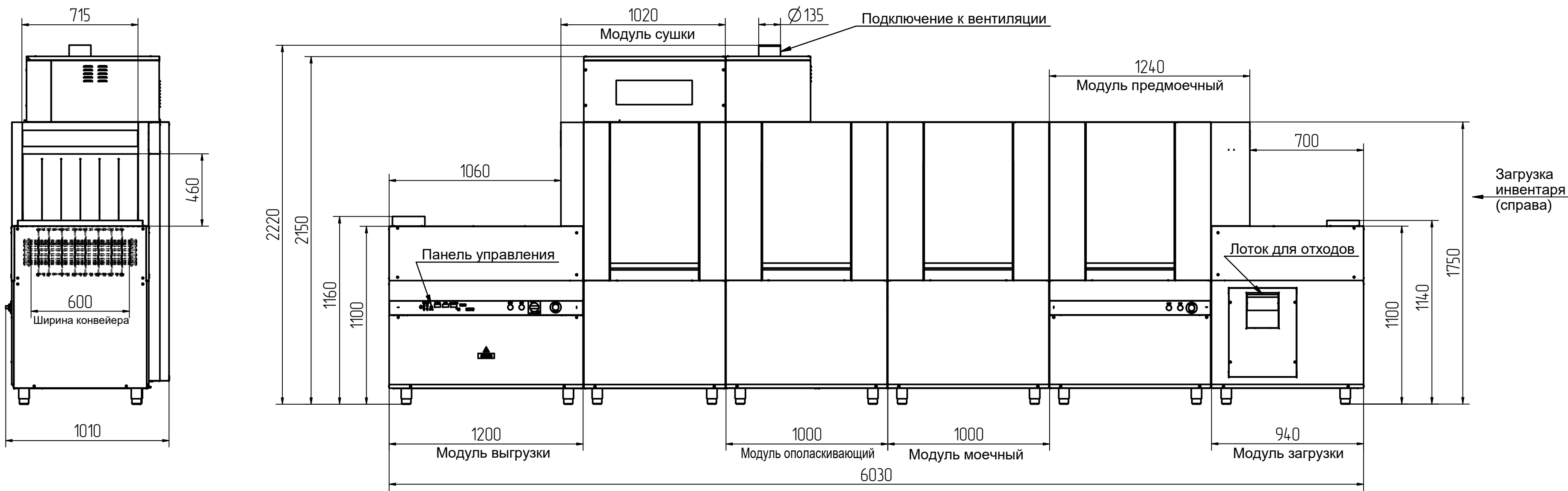
Изображение машины МПТ-3000К правого исполнения
