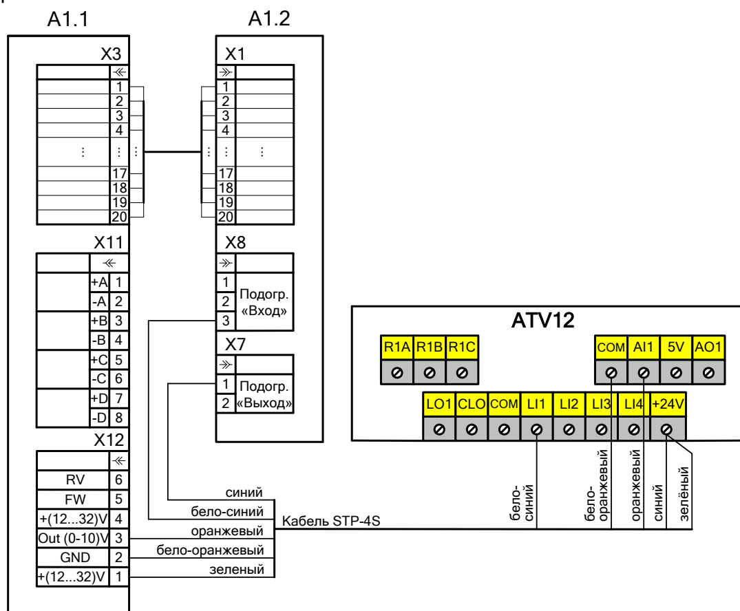
Рис. 14. Схема подключения частотного преобразователя ATV12
