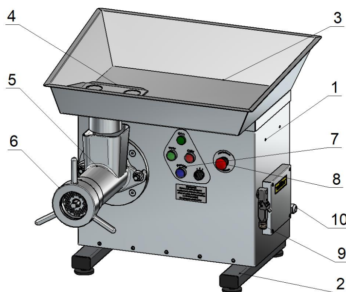
Рис. 1 Устройство мясорубки
