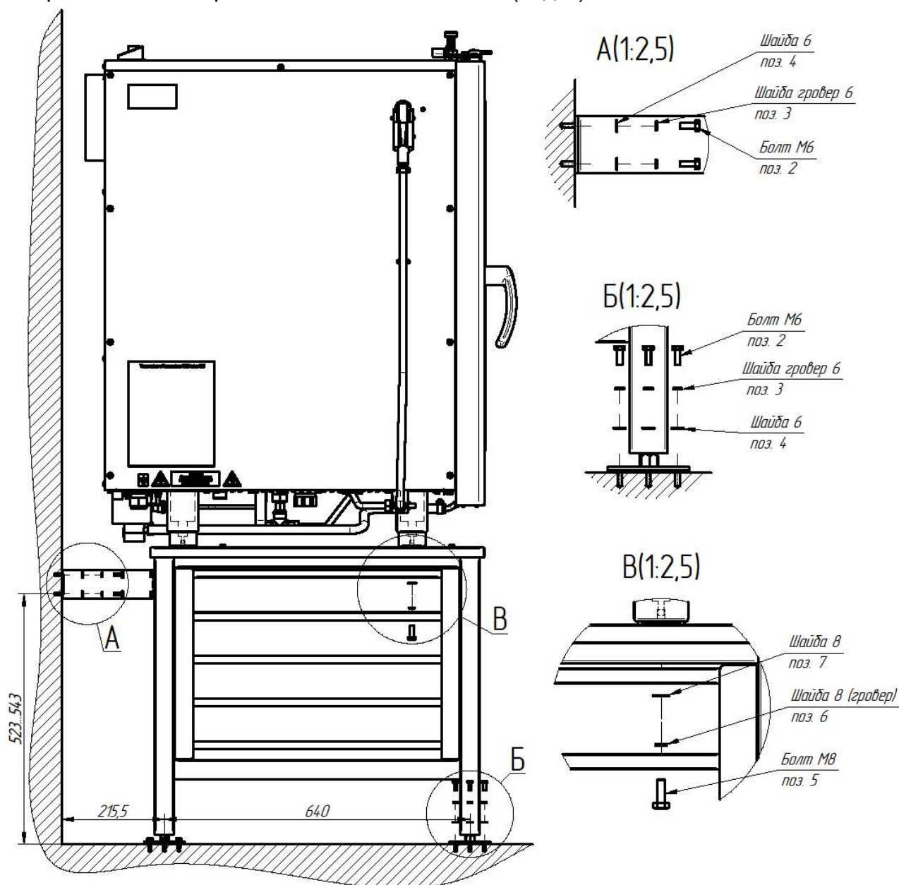
Установка подставки вид сбоку
