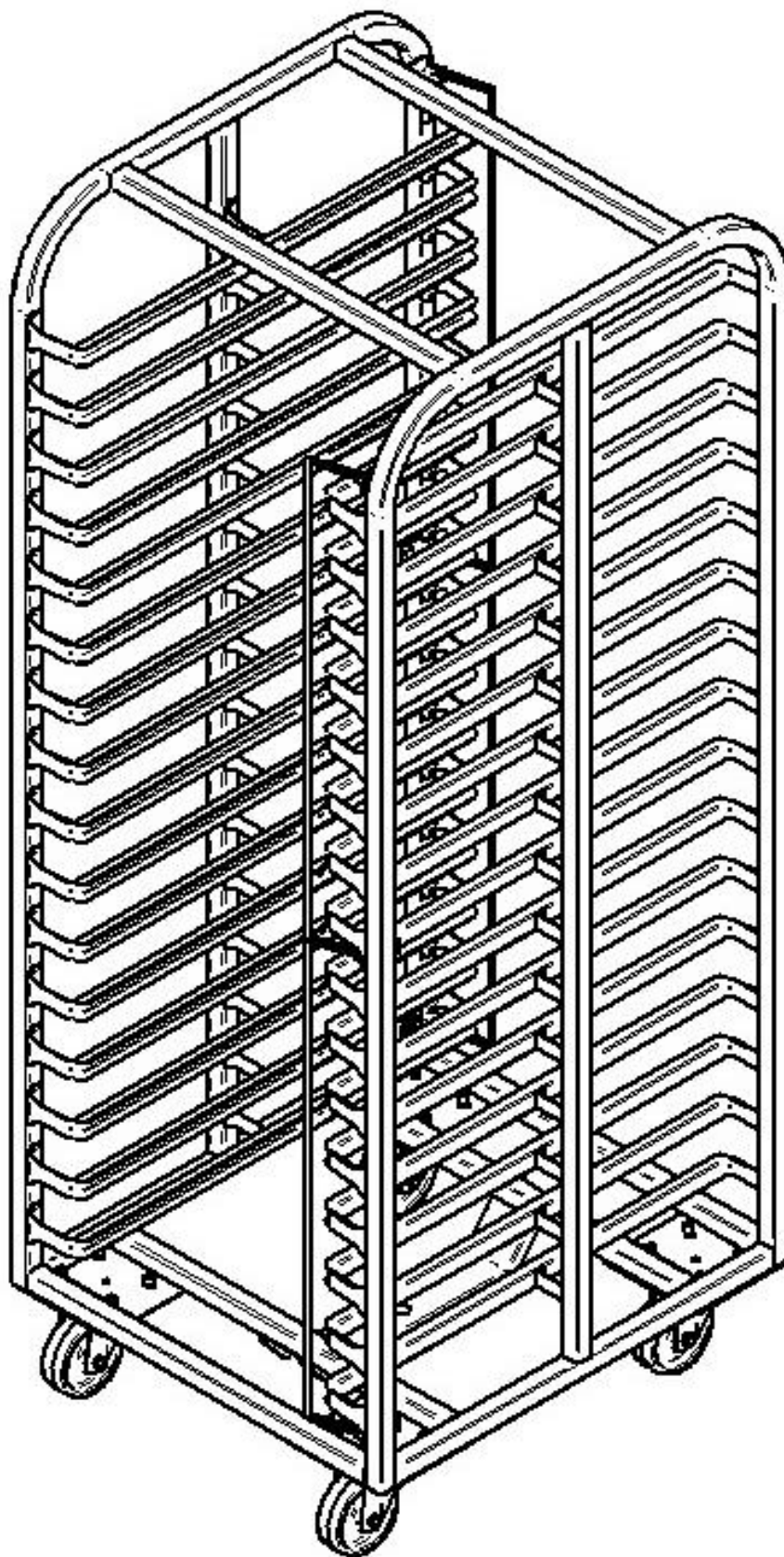
Рис.1 Общий вид ТШГ-16-01 универсальной
